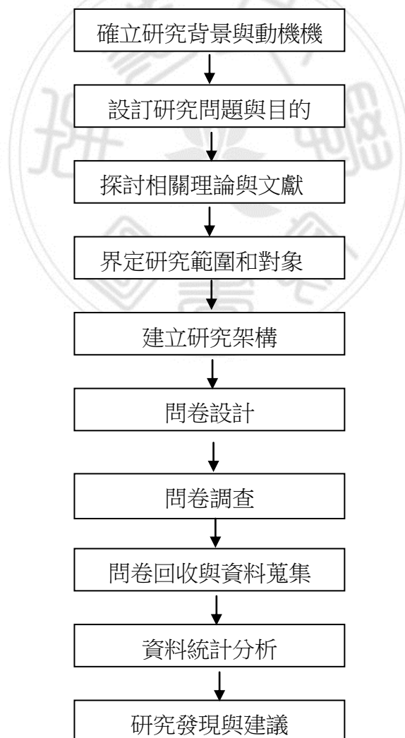
圖 1.1 研究流程
