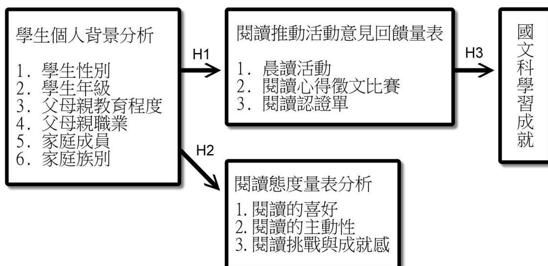
圖 3.1 研究架構圖
