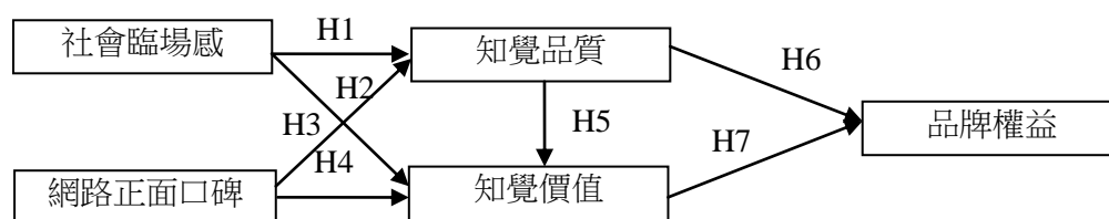
圖 1 研究模型
