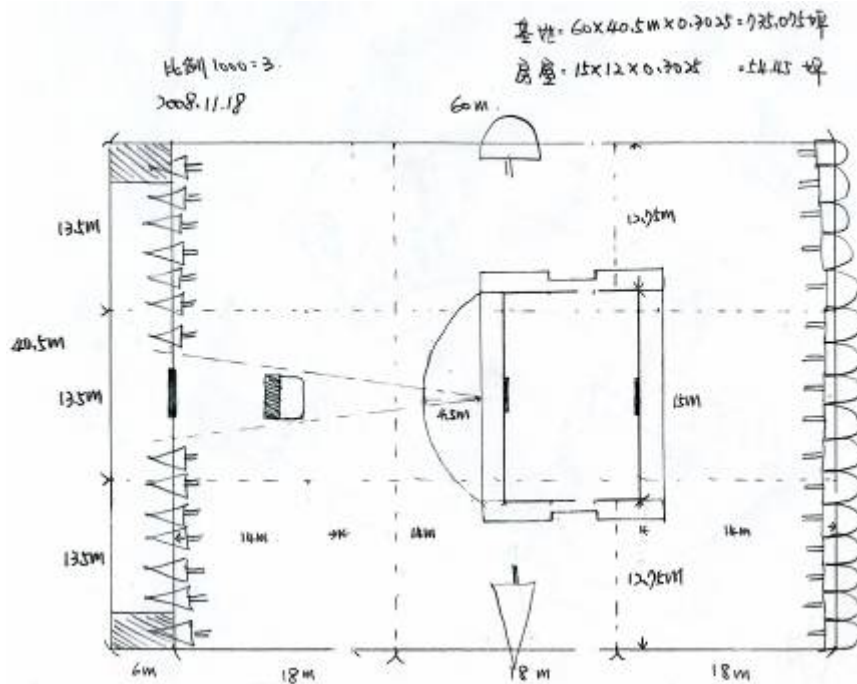
圖 4-1-16：理想建築外局平面圖 筆者自繪
