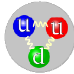
圖 2-1-2：質子的夸克組成
