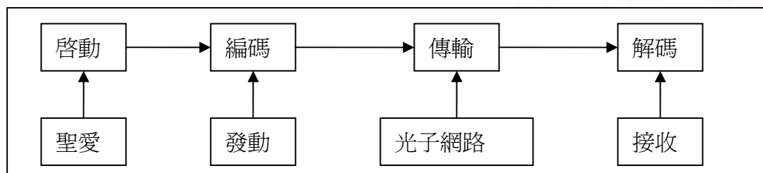
圖 2-2-5：光子密碼傳送流程 筆者自繪
