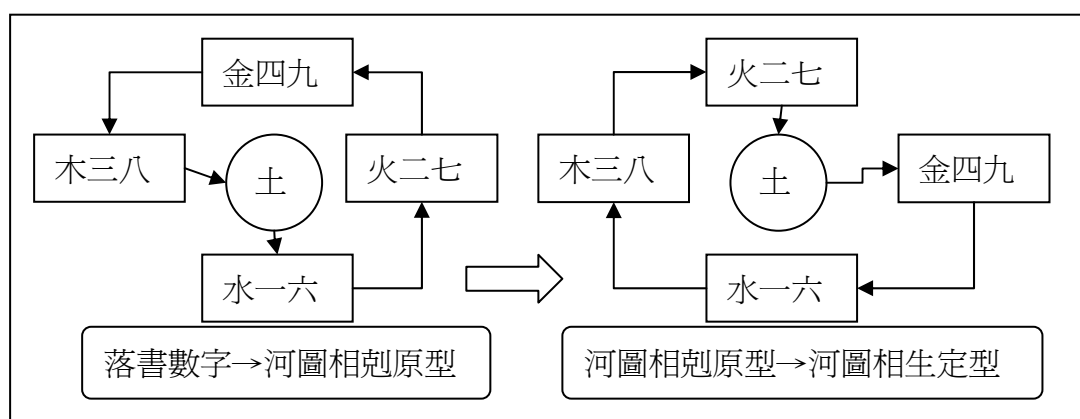
圖 5-1-13：洛書演變河圖原型到河圖定型 筆者自繪
