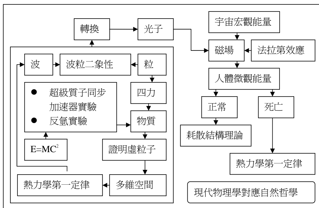
圖 2-1-4：現代物理學解釋能量轉換理由 筆者自繪
