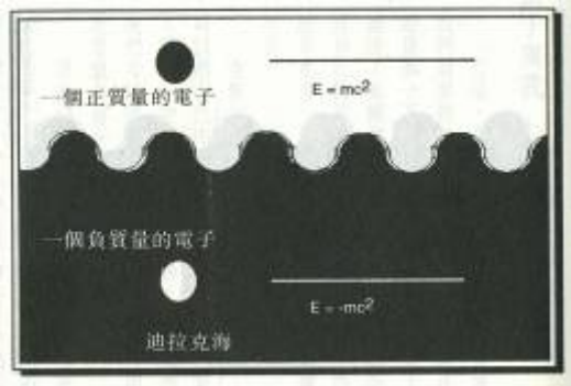
圖 2-3-4：迪拉克海 (Fred Alan Wolf 1999p.135) (左)
