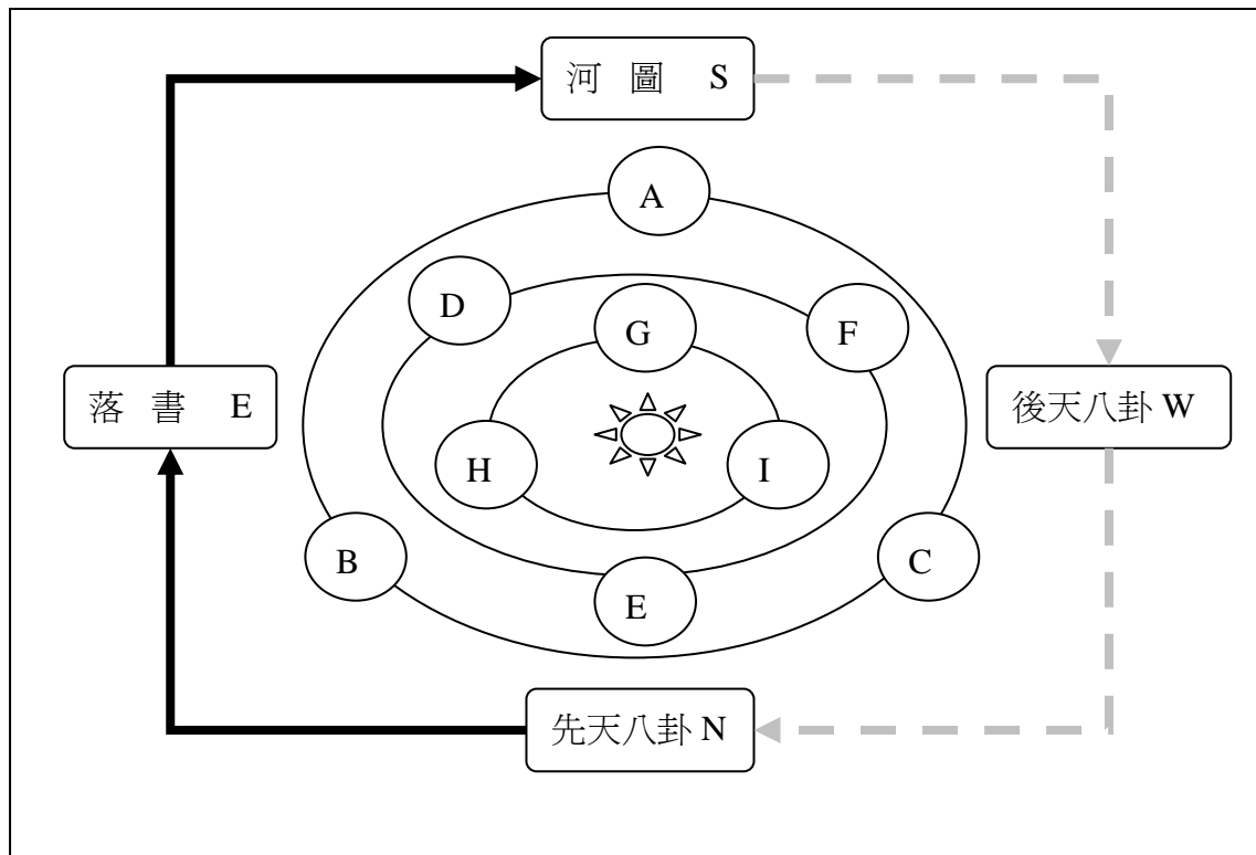
圖 6-2-1：宇宙圖示系統圖 筆者自繪
