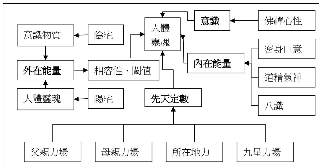
圖 5-1-7：人和四力之關聯圖 筆者自繪
