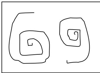
圖 2-3-6：原初粒子（參考王大有 2006p.44 筆者自繪）（左）
