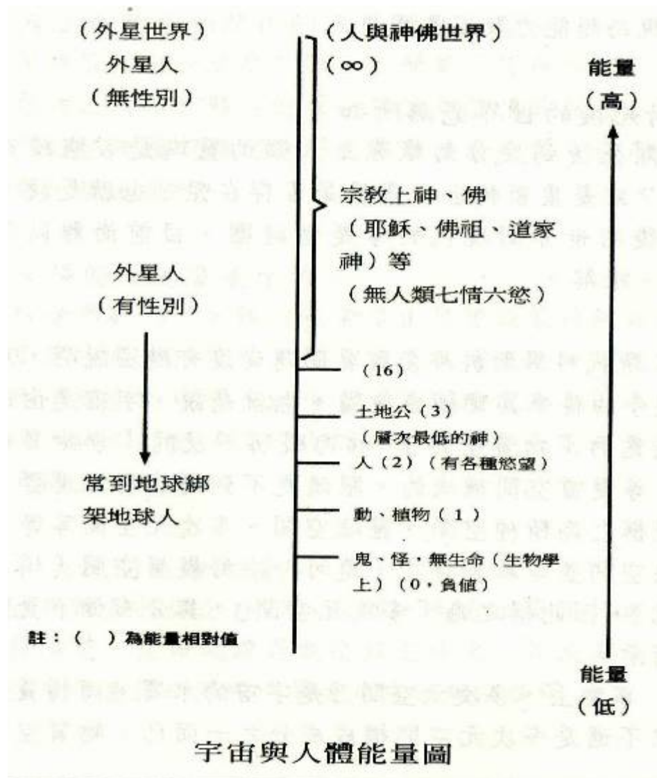
圖 2-1-5：宇宙與人體能量圖（江晃榮 2007p.138）
