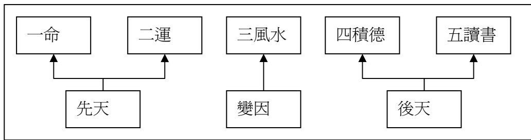
圖 1-1-3：命運結構 筆者自繪
