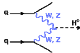
圖 2-1-3：希格拉斯粒子
