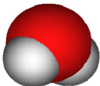
圖 2-2-6：水分子圖 (左)
