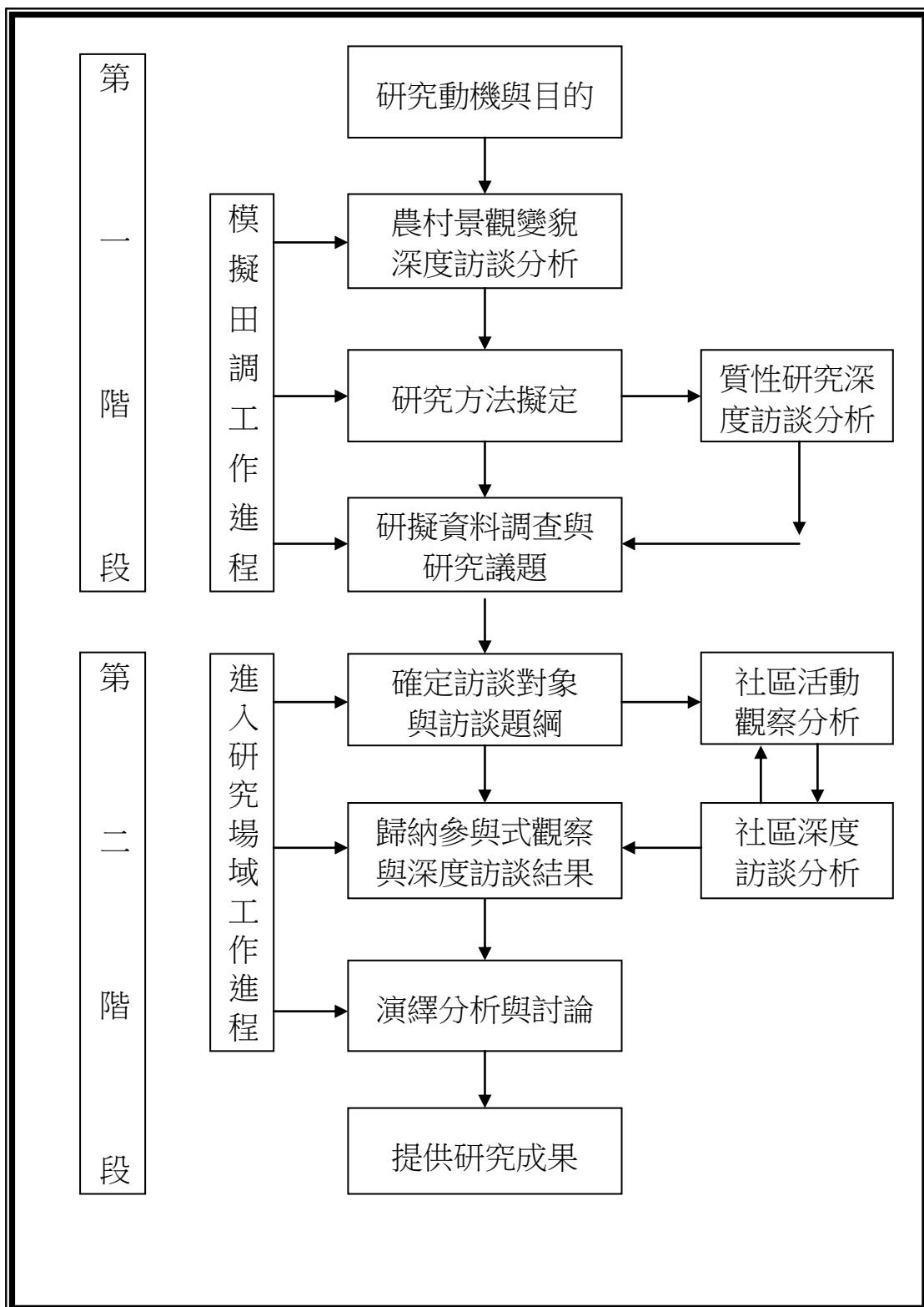
圖 1.4.1 研究流程圖
